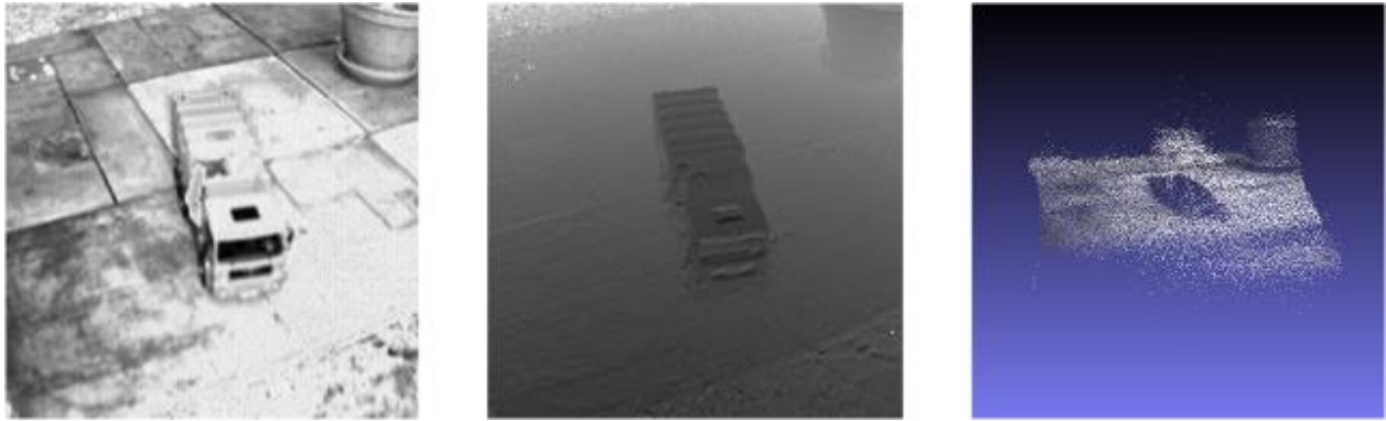
Abb. 16: Passives Intensitätsbild, Entfernungsbild und texturierte 3D-Punkt wolke.
