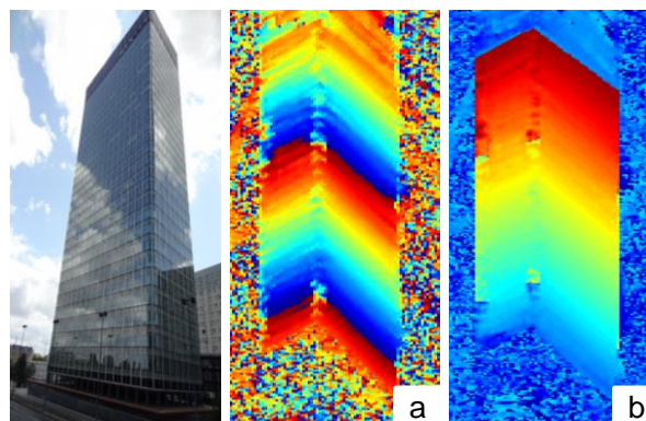
Abb. 2: Phase Unwrapping auf TanDEM-X Phasendaten; a) gefiltertes Phasenbild; b) abgewickelte Phase
