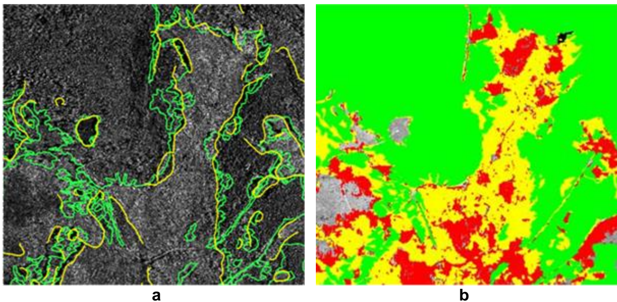
Abb. 6: Ergebnis der Wandrandextraktion (a) - manuell (grün) und automatisch (gelb), Überlagerung der multitemporalen Waldflächen (b) - Orthophoto (rot, 2007), RapiEye (gelb, 2011) und TerraSAR-X (grün, 2011)
